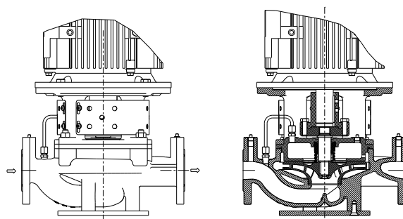
ESL 25-32-40-50
