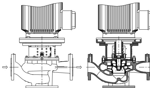
ESL 65-80-100
