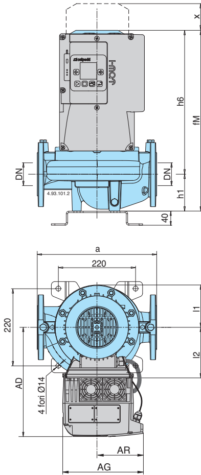
Flanges PN 10, EN 1092-2
