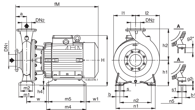
Flanges EN 1092-2
